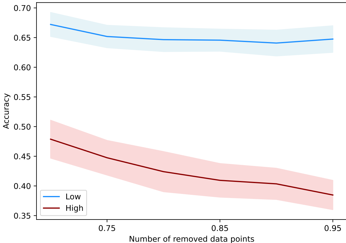
DataAttrOpt(10000, 0.03, 15, inf, +b, alpha=1.0) - pol
